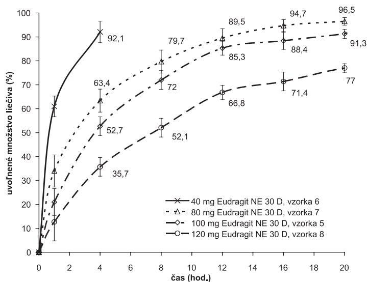
Obr. 4. Liberačné profily metformíniumchloridu z matricových tablet v závislosti od množstva polyméru
