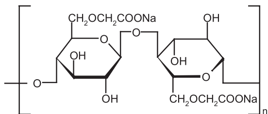
Obr. 5. Strukturní vzorec sodné soli karmelosy
