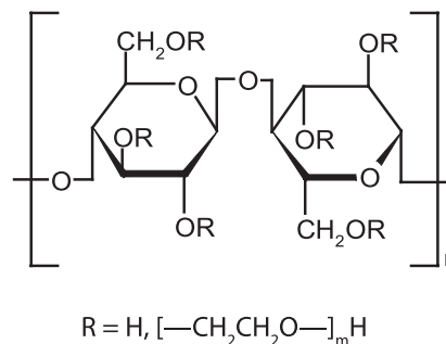
Obr. 6. Strukturní vzorec hyetelosy
