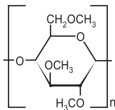
Obr. 2. Strukturní vzorec methylcelulósy
