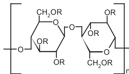
Obr. 3. Strukturní vzorec hydroxypropylcelulósy
