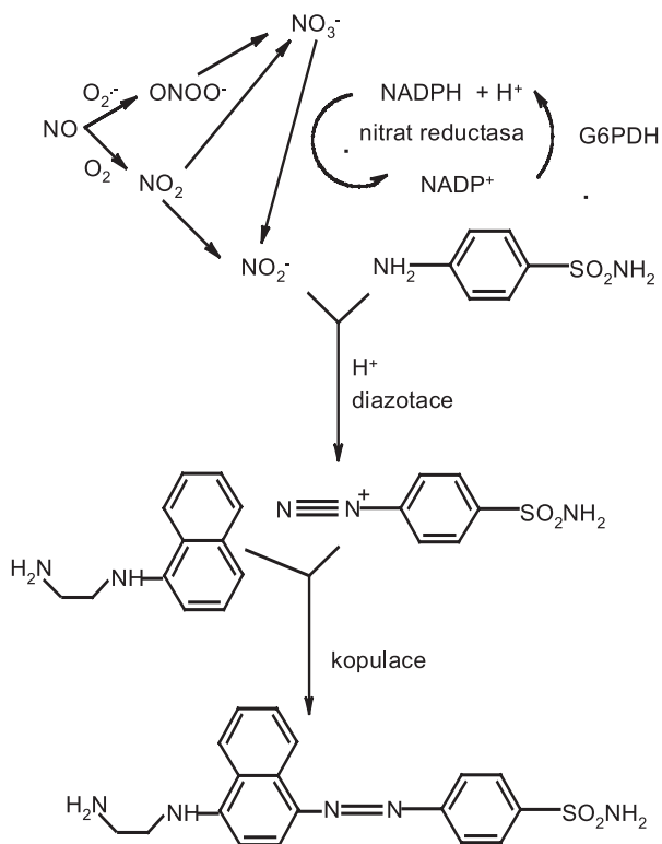
Obr. 1. Griessova reakce
