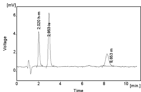
Obr. 7. Chromatogram patientského vzorku – koncentrace metoprololu (m) 84,8 ng/ml a koncentrace \alpha -hydroxymetoprololu (h-m) 162,7 ng/ml
