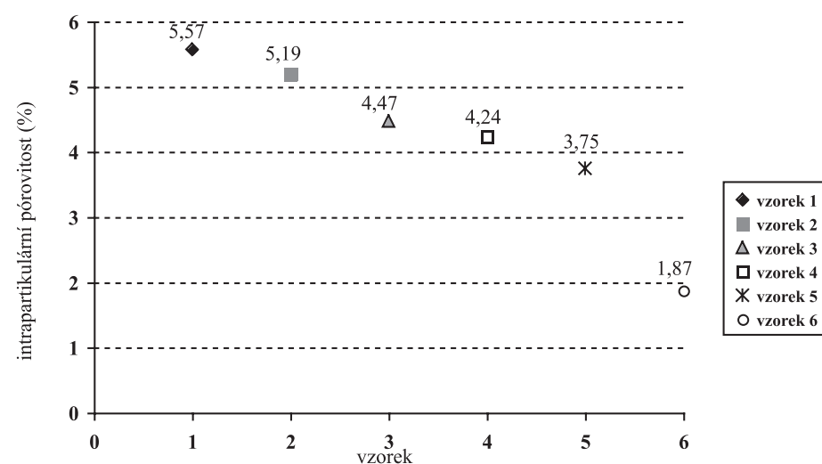
Obr. 4. Intrapartikulární pórovitost
