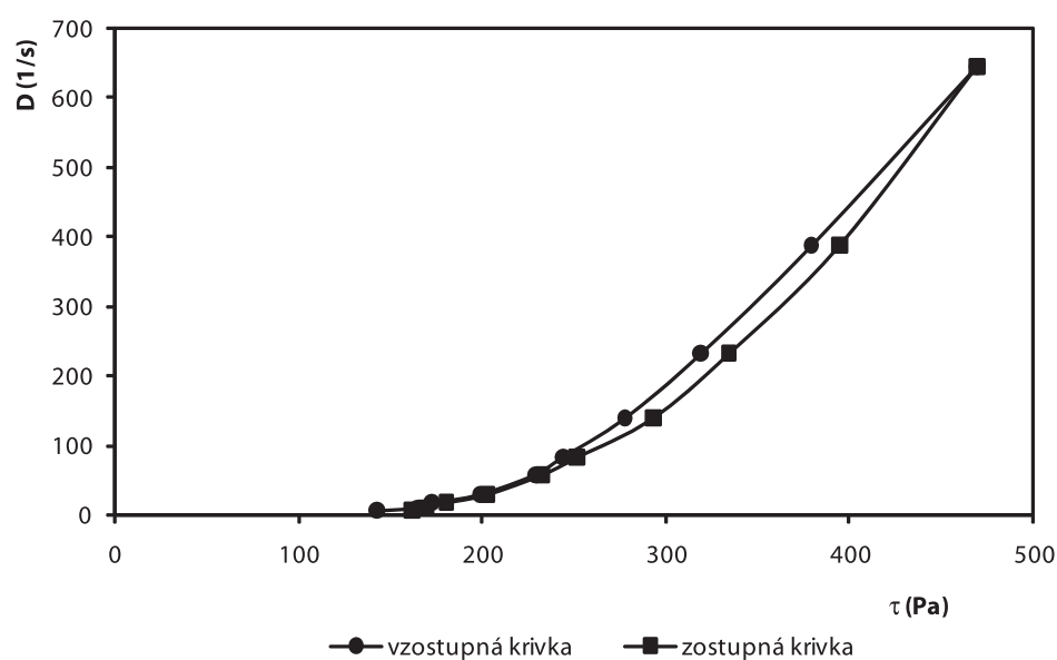
Obr. 3. Toková krivka hydrogélu vzorky č. 8 po 28 dňoch
