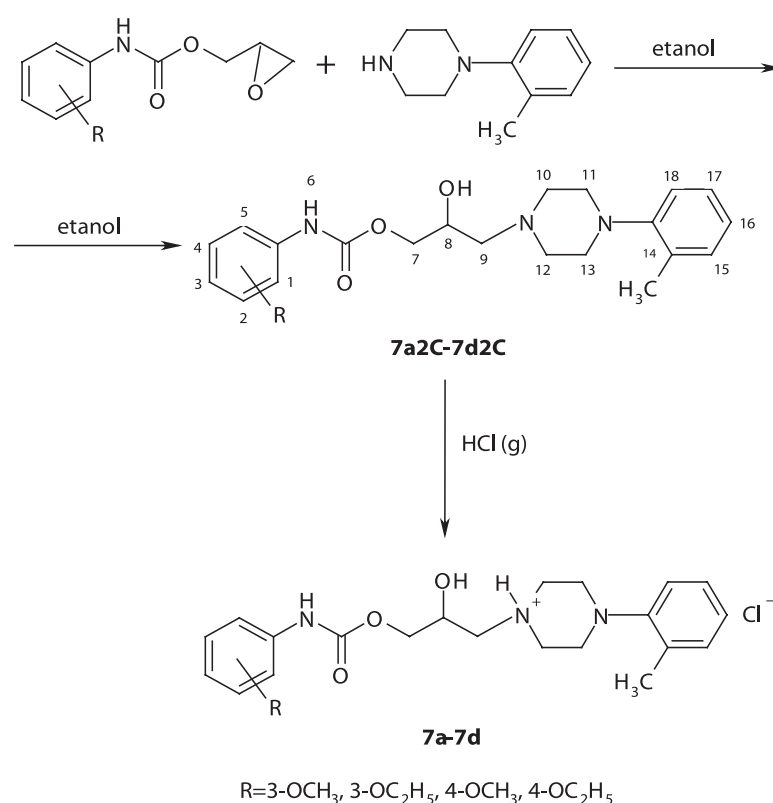
Obr. 1. Schéma prípravy 1-[3-(Y-alkoxyfenylkarbamoyloxy)-2-hydroxypropyl]-4-(2-metylphenyl)piperazíniumchloridov ( 7a-7d ); číslovanie skeletu zlúčenín 7a2C-7d2C z hľadiska ^1\text{H-NMR} spektrometrie
