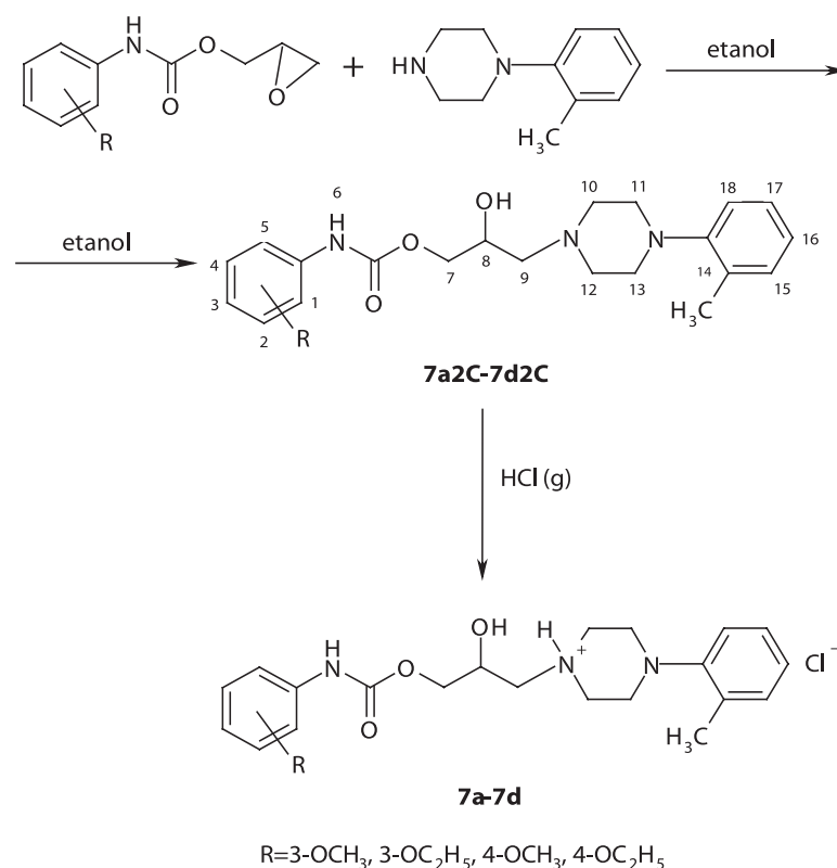
Obr. 1. Schéma prípravy 1-[3-( Y -alkoxyfenylkarbamoyloxy)-2-hydroxypropyl]-4-(2-metylphenyl)piperazíniumchloridov ( 7a-7d ); číslovanie skeletu zlúčenín 7a2C-7d2C z hľadiska ^1\text{H-NMR} spektrometrie
