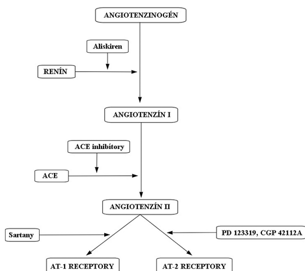
Obr. 1. Systém RAAS
