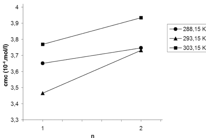
Obr. 5. Závislost kritické micelové koncentrace od počtu atomů uhlíku v n-alkanole (n) v roztoku pentakainiumchloridu při teplotách 288,15 K, 293,15 K a 303,15 K
