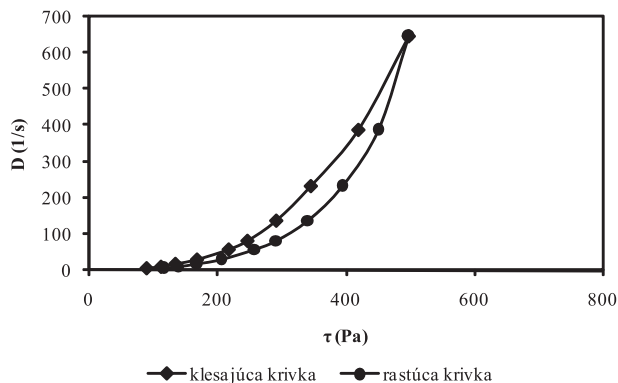
Graf 3. Toková krivka hydrogélů s obsahom: 2,5 % CHIT (typu B) + 5 % SAL + 5 % GLY
