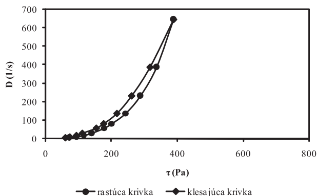
Graf 2. Toková krivka hydrogélů s obsahom: 2,5 % CHIT (typu A) + 5 % SAL + 5 % GLY
