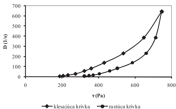
Graf 1. Toková krivka hydrogélů s obsahom: 1 % CAR + 5 % SAL + 20 % GLY
