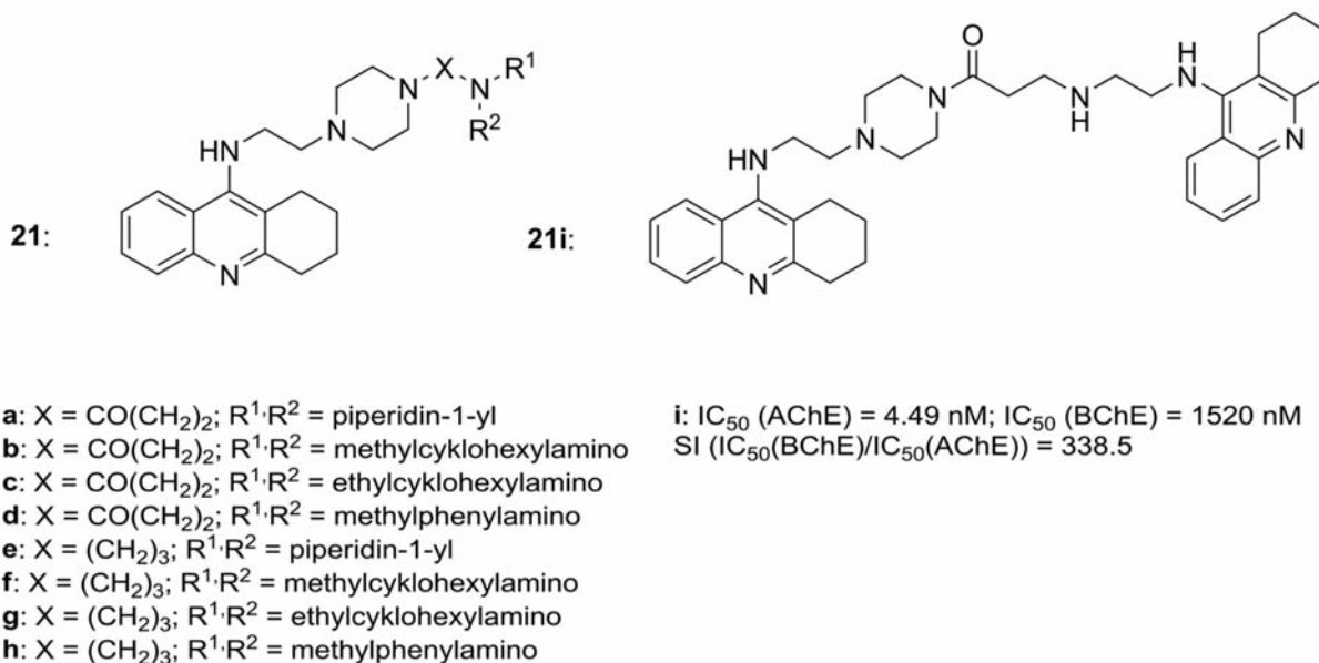
Obr. 21. Takrin-piperazinová série
