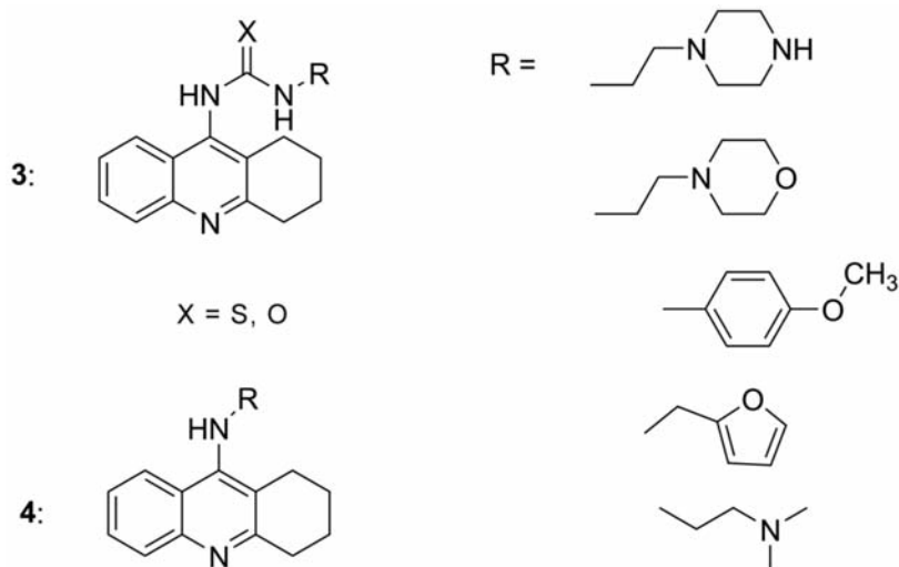
Obr. 3. Takrinová analoga připravená substitucí v poloze 9
