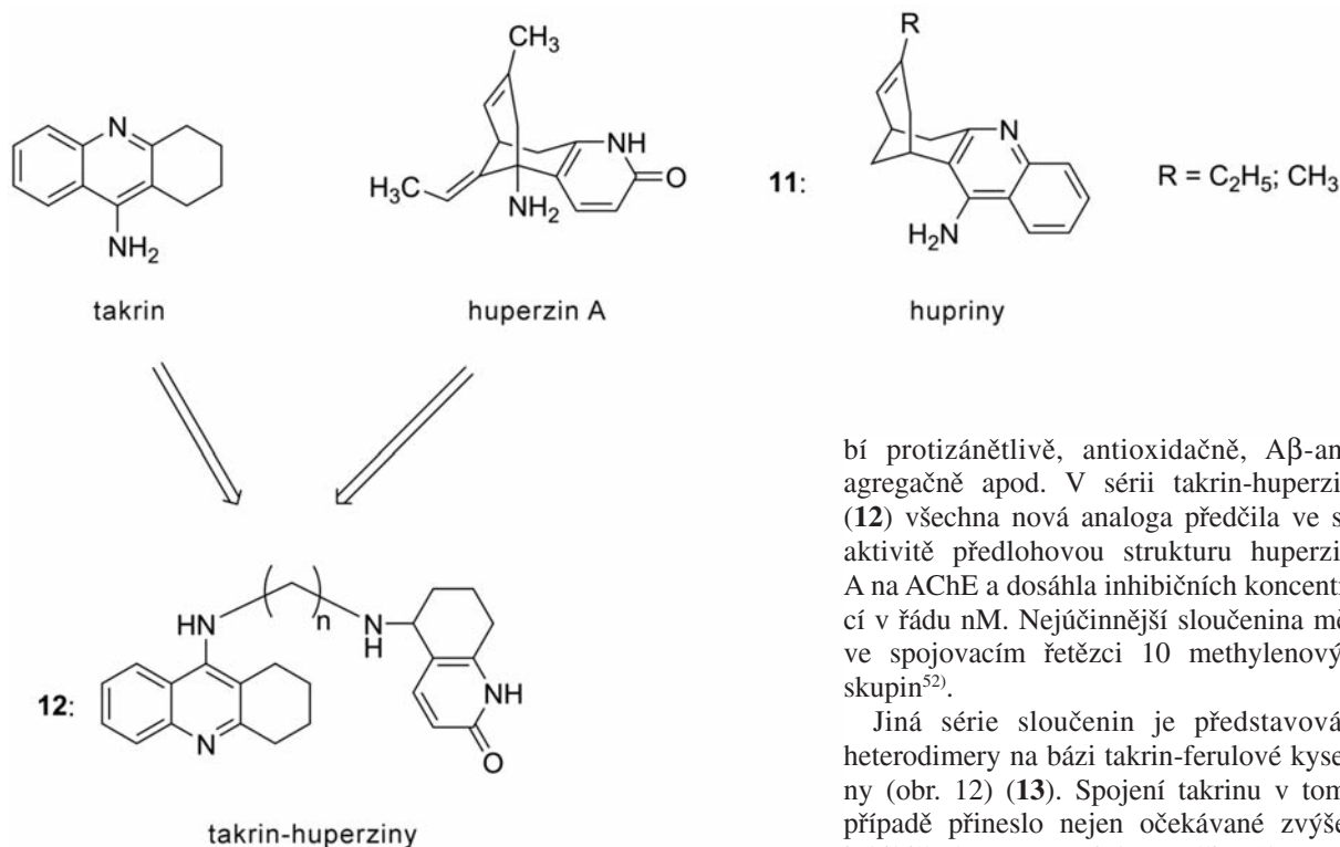
Obr. 11. Takrin-huperzinové deriváty a hupriny
