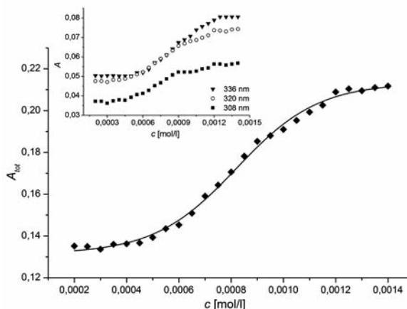
Graf 1. Závislosť súčtu absorbancií hlavných pyrénových pík ( A_{\text{tot}} ) od koncentrácie ( c ) látky XXIX Z vo vodnom prostredí pri 25 °C
