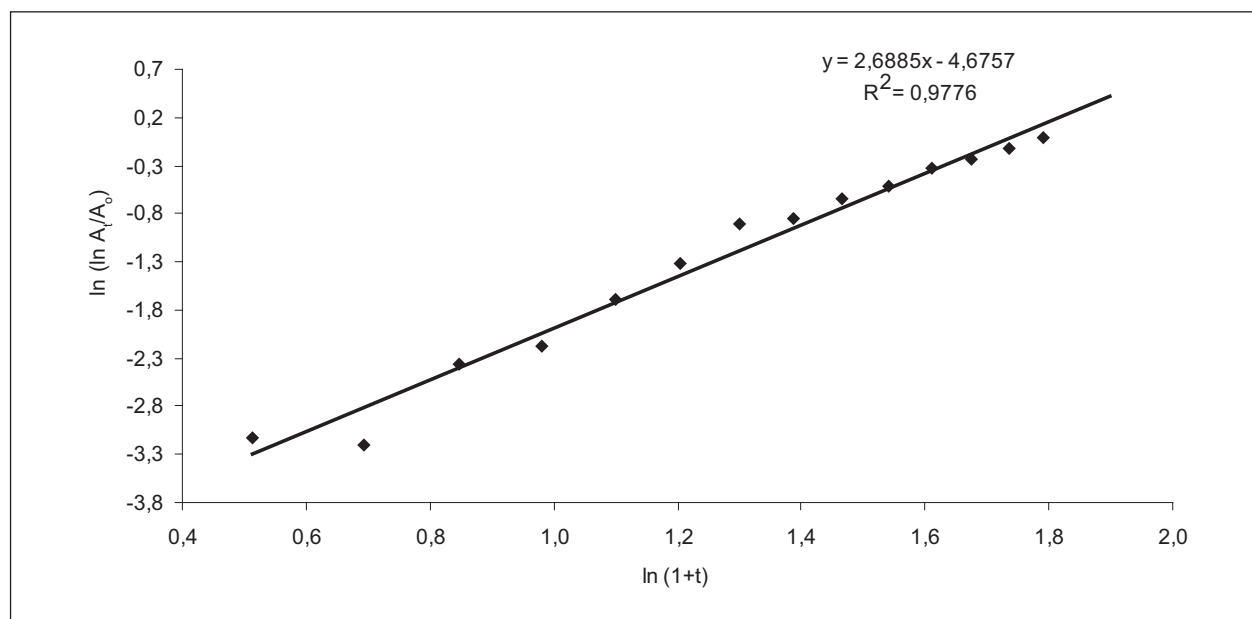
Graf 2. Vyhodnotenie neizotermického testu heptakaíniumchloridu v rozsahu teplôt 40–82 °C v prostredí vodno-etanolového roztoku hydroxidu sodného c = 0,1 \text{ mol/l}
