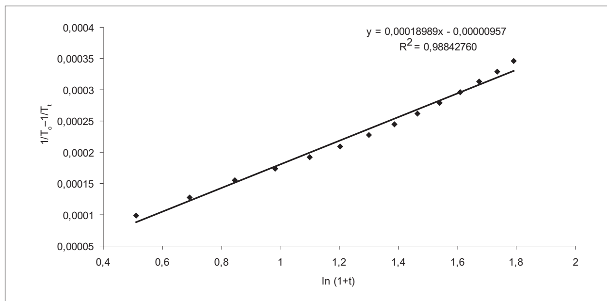
Graf 1. Rast teploty ( K^{-1} ) v rozsahu 40–82 °C pre heptakaíniumchlorid
