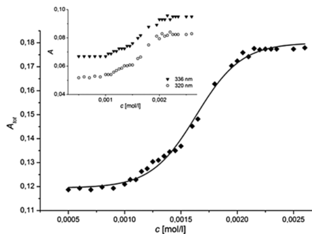
Graf 5. Závislosť súčtu absorpcií hlavných pyrénových pík ( A_{\text{tot}} ) od koncentrácie látky H34 ( c ) v 3 mol/l etanolovom prostredí pri 25 °C
