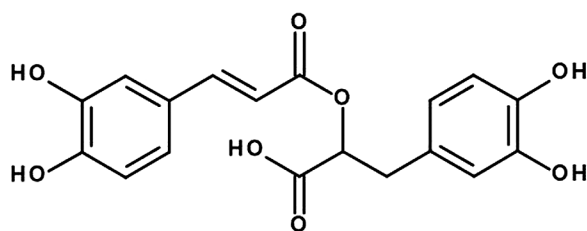
Obr. 1. Kyselina rozmarínová
