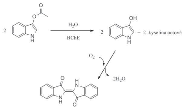
Obr. 4. Stanovení aktivity cholinesteras za využití indoxylacetátu jako fluorogenního a chromogenního substrátu. Reakční schéma je upraveno z citovaných prací 61, 62 .
