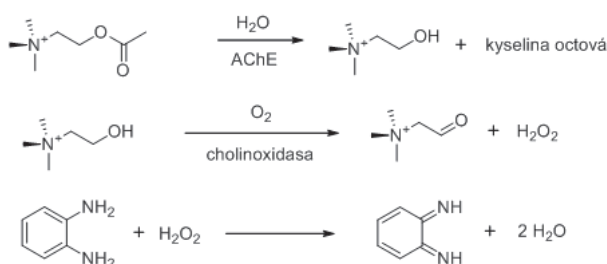
Obr. 3. Využití cholinoxidasy při stanovení aktivity AChE. Znárodně je i použití chromogenního substrátu reagujícího se vznikajícím peroxidem vodíku. Reakční schéma je upraveno z citovaných prací 61, 62 .
