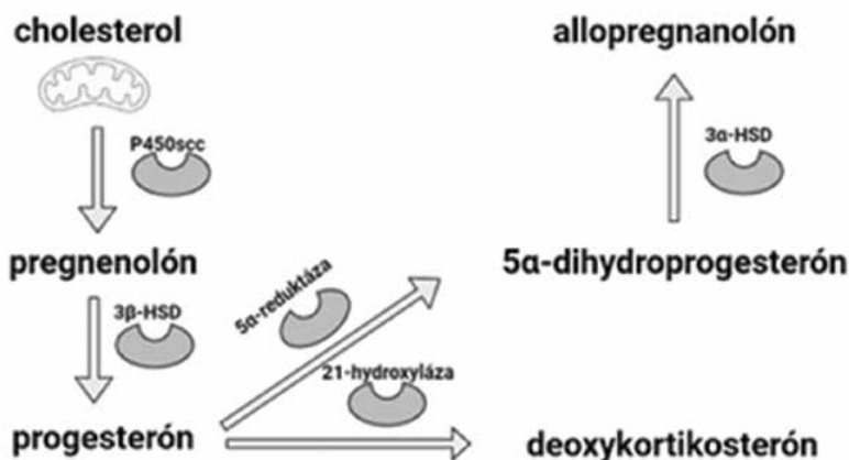
Obr. 1. Enzým P450scc štiepi cholesterol vo vnútornej mitochondriálnej membráne na pregnanový steroid pregnenolón. Ďalším štiepením pregnenolónu vznikajú hlavné steroidné metabolity s hypnotickým a anxiolytickým účinkom, konkrétne progesterón (cez enzým 3 \beta -HSD), deoxykortikosterón (štiepením progesterónu 21-hydroxylázou) a allopregnanolón (5 \alpha -reduktáza štiepi progesterón na 5 \alpha -dihydroprogesterón a ten sa následne štiepi pomocou enzýmu 3 \alpha -HSD na allopregnanolón).
