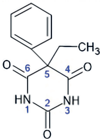
Obr. 1. Struktura fenobarbitalu (s označením pozic na pyrimidinovém skeletu)
